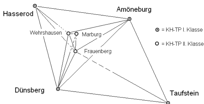
Abb. 5: Detailnetz bild zur kurhessischen Haupttriangulation im Raum Marburg
